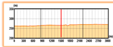
第1区縦断面図 競技場～興譲館高校西 3.0Km
