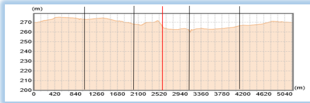
第3区 縦断面図
