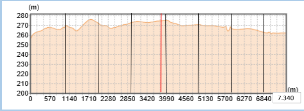
第5区 縦断面図
